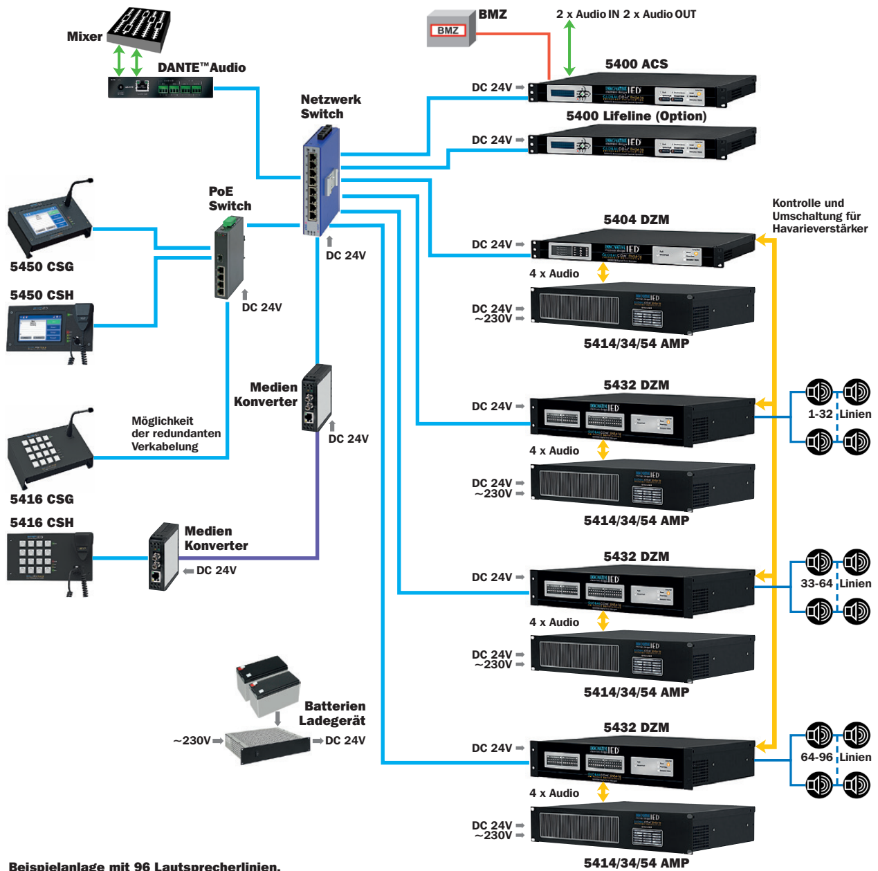
Beispielanlage mit 96 Lautsprecherlinien. Leistung zwischen 1200 Watt und 6000 Watt (abhängig von verwendeten Verstärkern).
